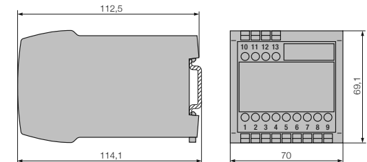
Bild 2. Gehäuse P13/70 auf Hutschiene (35 x 15 mm oder 35 x 7,5 mm, nach EN 50 022) aufgeschnappt.
